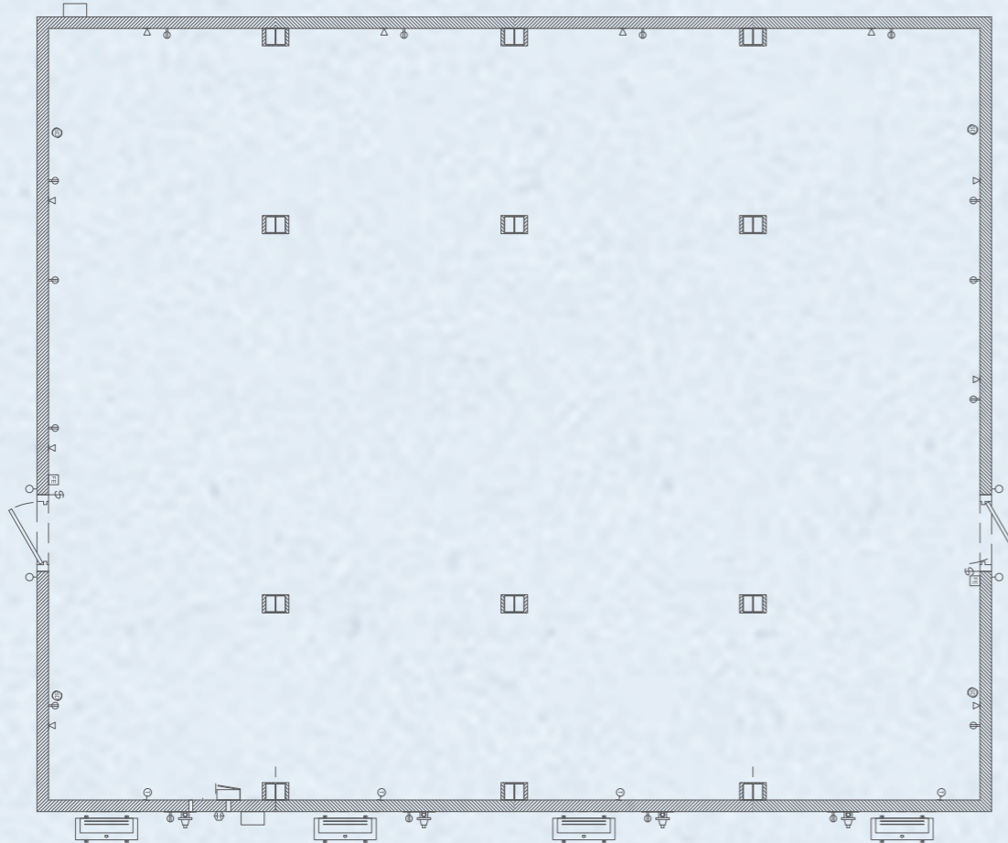
48 OP 48W X 40L X 11H OPEN PLAN
